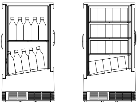
500mlPET 2段 350ml缶 4段 (オプション棚1枚追加仕様の場合)
