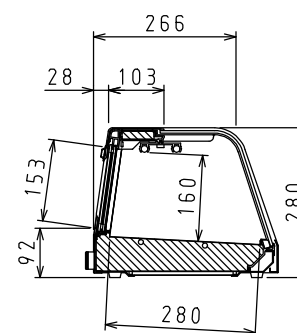
側面断面図
