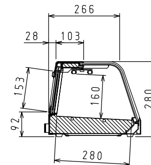
側面断面図
