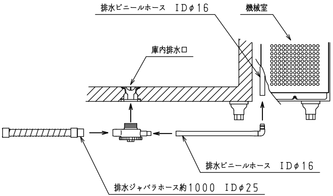
排水部詳細
