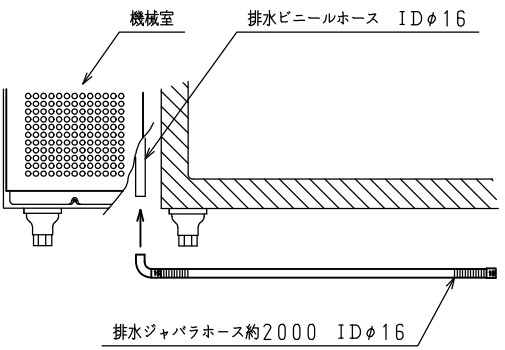
排水部詳細
