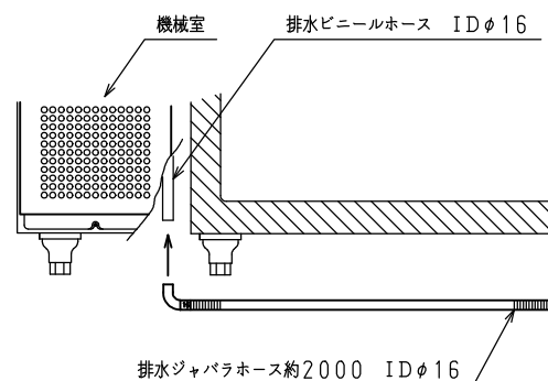
排水部詳細
