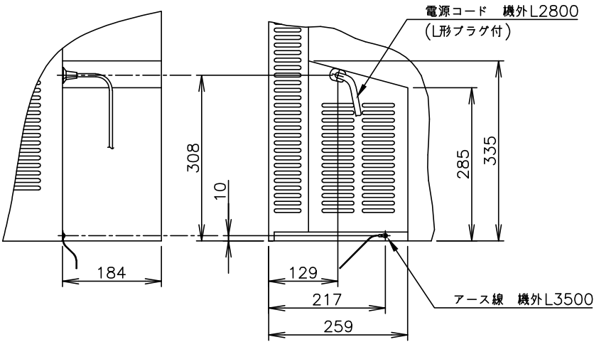
B矢視図(1/10)
