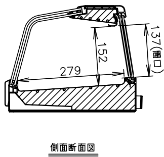
側面断面図
