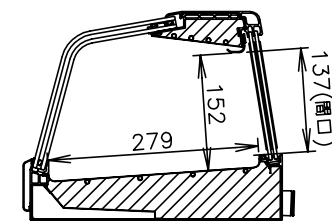
側面断面図
