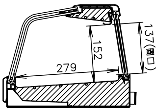
側面断面図
