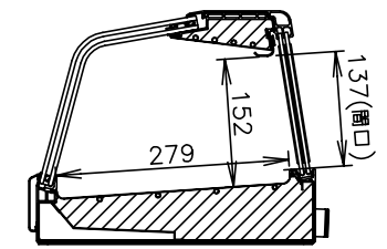
側面断面図
